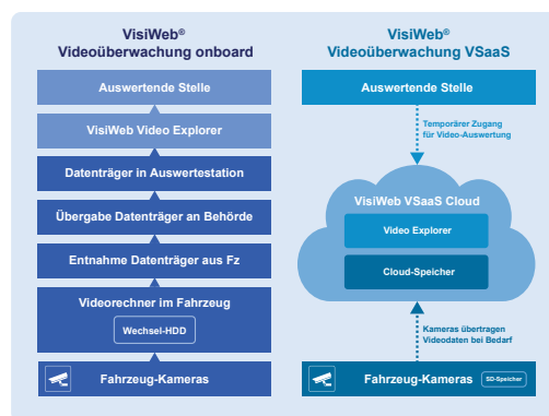
Zur Auswertung des Videomaterials erhält die Behörde einen sicheren, temporären Zugang auf die VisiWeb VSaaS Cloud.
